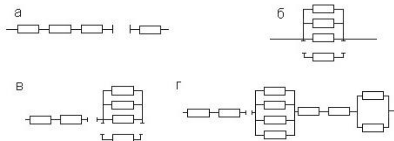
Рисунок 5 Схемы соединения элементов системы газоснабжения
